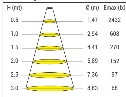
QDR 2 60x60 CW 24W 24V DC IP44
