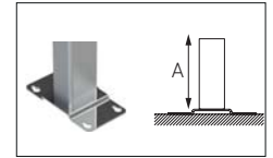
34: Uzatma parçası A=5cm 35: Uzatma parçası A=10cm 36: Uzatma parçası A=20cm
